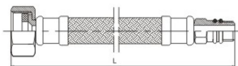
KLOE813A F1/2"x M10*1
