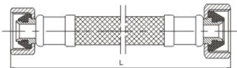
KLOE8223 F1/2"C×F1/2"
