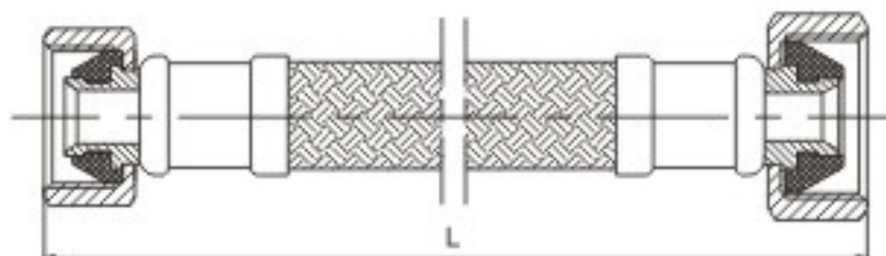
KLOE8123 F1/2"C×F1/2"
