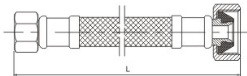
KLOE8213 F1/2"×F3/8"C
