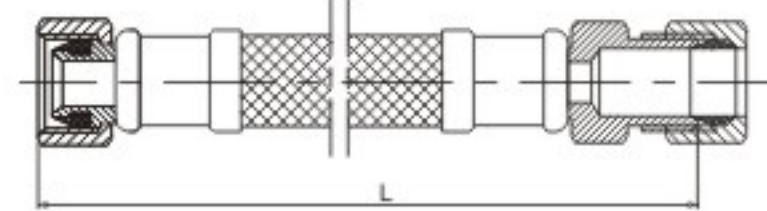
KLOE8219 M3/8"C×F3/8"C
