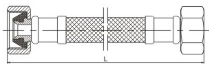
KLOE8233 F1/2"×F1/2"
